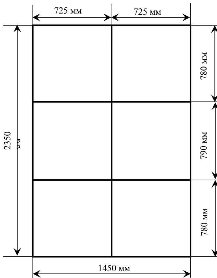
Схема на прозорец по позиция № 2
