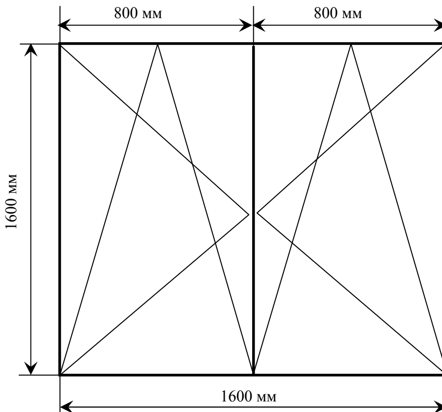
Схема на прозорец по позиция № 1
