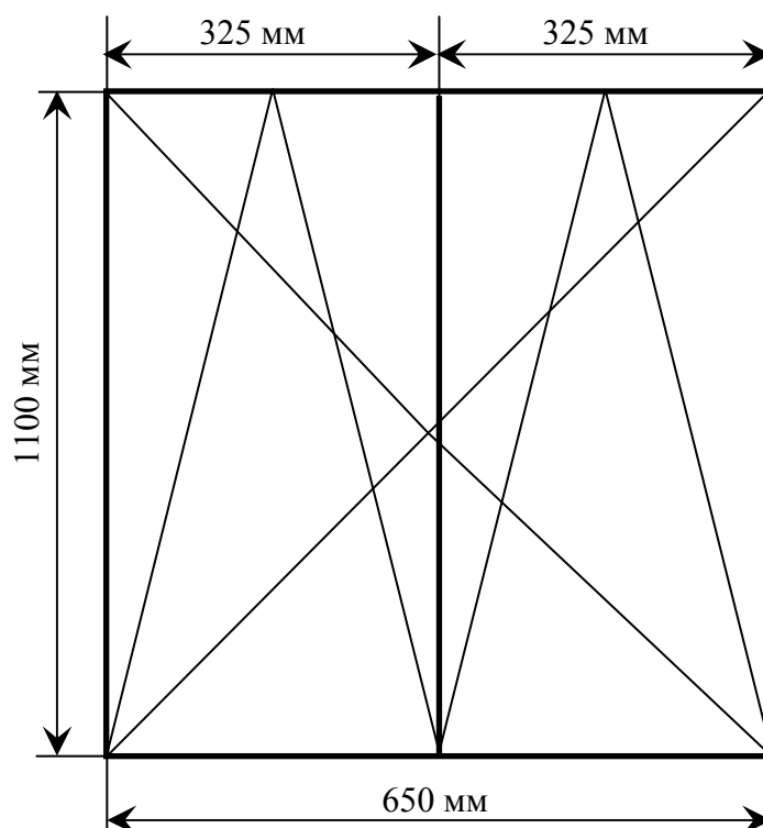
Схема на прозорец по позиция № 3
